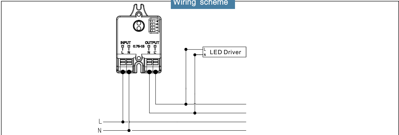
Wiring scheme
